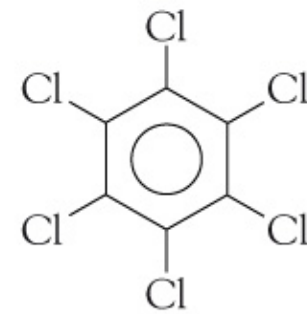
hexachlorobenzene (HCB)
