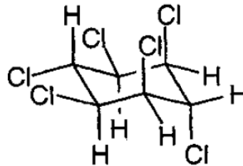
lindane
